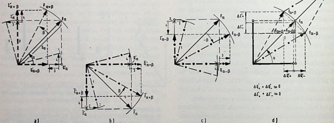
Fig. 16. Kleurenfout-compensatie bij het PAL-systeem. Twee lijnen worden achter de beide synchroon-demodulators I' en Q' opgeteld (of in het oog):
