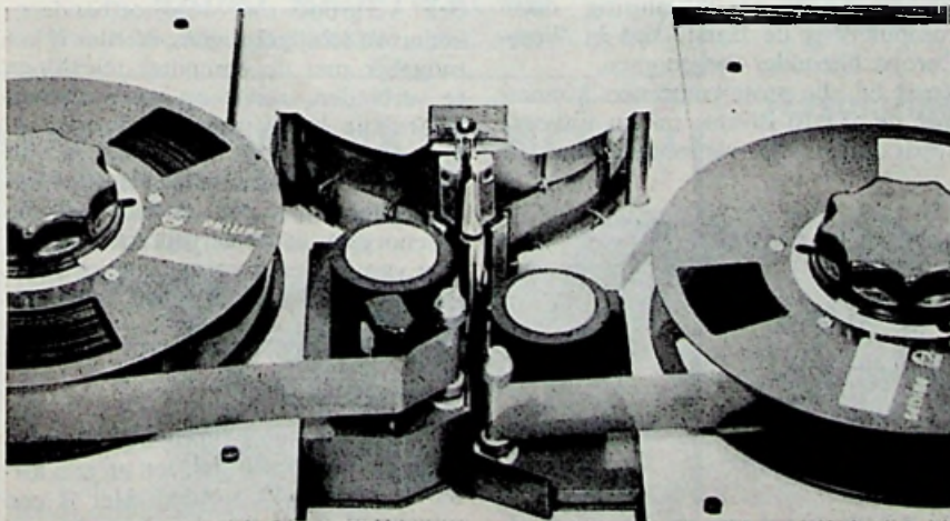
Dichtbijopname van de trommel en het bandtransportmechanisme van de Philips video-recorder. De aandrukrollen spannen de band.
