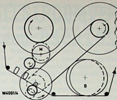
Fig. 4. Bandloop en aandrijving van de Optacord 500.
