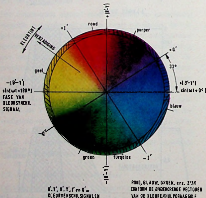
Fig. 5. Kleurencirkel, die de stand van de hulpdraaggolf- vector voorstelt in het vlak van de hulpdraaggolf. Bij elke hoek behoort een kleurtint. De vector-amplitude bepaalt de kleurverzadiging.
