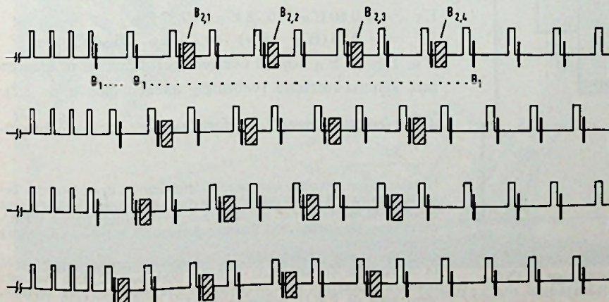
Fig. 25. Kleursynchroon- en identificatie-signalen in vier na elkaar volgende rasters. (Hierna wordt de situatie herhaald.)
