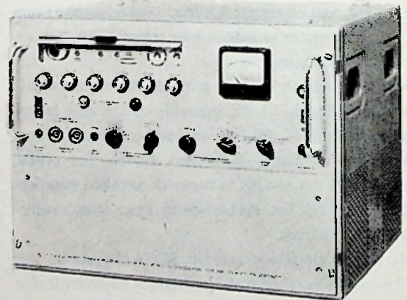
MEET-DEMULATOR, TYPE AMF Naar keuze voor band I, III of IV/V
