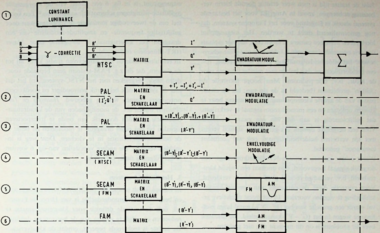
Fig. 6. Blokschema van het NTSC-systeem en enige van zijn varianten (alle niet getekende blokjes gelden als bij NTSC; de coëfficiënten bij de klein verschilsignalen zijn niet aangegeven).
