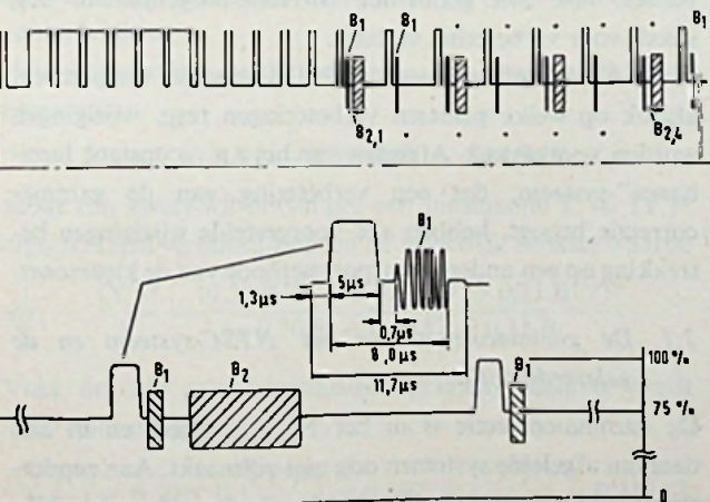
Fig. 3. Kleursynchroon-sig-naal (Burst) en de identificatie-impulsen bij het PAL-systeem, welke verderop in dit artikel worden toegelicht.
