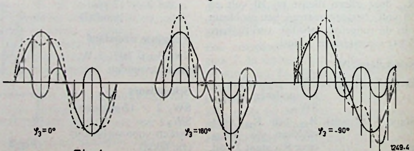
Fig.4 GRONDTTOON + 3 e HARMONISCHE
