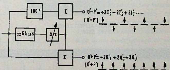
Fig. 24. SECAM-O'-P'-systeem, gemoduleerd in de PAL-decoder met looptijd-demodulator.
