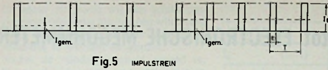
Fig. 5 IMPULSTREIN
