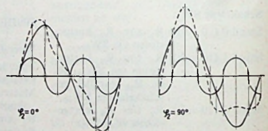
Fig.3 GRONDTTOON + 2 e HARMONISCHE
