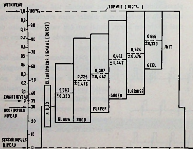
Fig. 26. Video-siginaal voor verzadigde kleurbalken met 75% amplitude van R' , G' en B' volgens de voorlopige NTSC-normalisatie in Duitsland.
