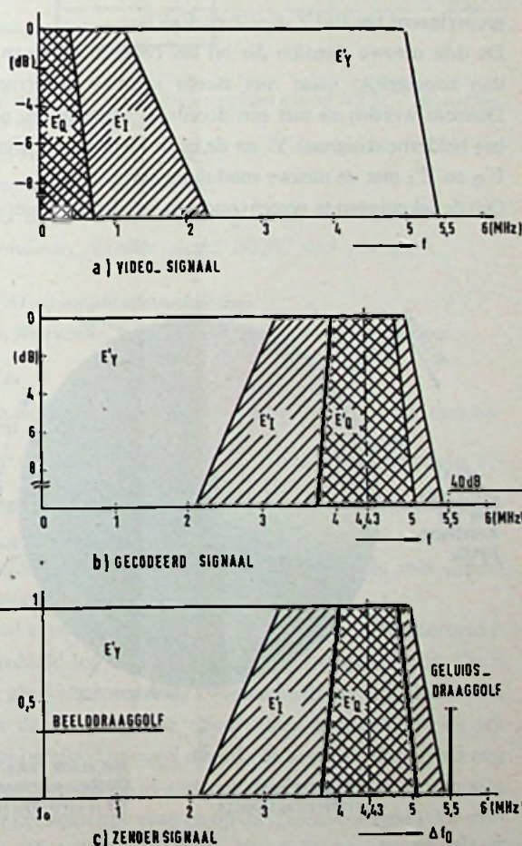
Fig. 4. Bandbreedten van het Y'- I'- en Q'-sig-naal in het NTSC-systeem voor 625 lijnen met een frequentie-afstand van 5,5 MHz tussen beeld- en geluidsdraaggolf.
