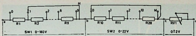
Schakeldeks gezien van achterzijde
