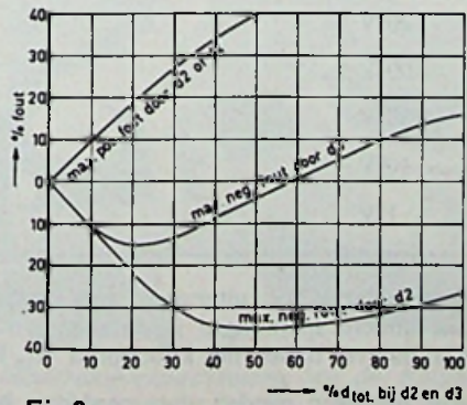
Fig. 9 INVLOED VAN d_2 en d_3 BIJ TOPMETER
