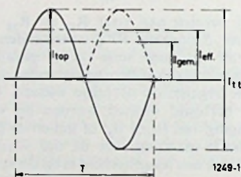
Fig.1 SINUSVORMIGE STROOM
