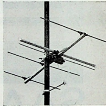
NORDESSA antenne voor TV-NOORDZEE van 3 tot 15 elementen
