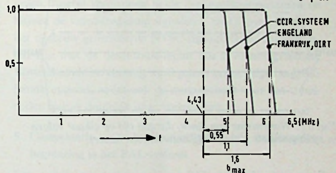
Fig. 12. De video-bandbreedte voor de drie genormaliseerde systemen met 625 lijnen in Europa voor band IV en V.
