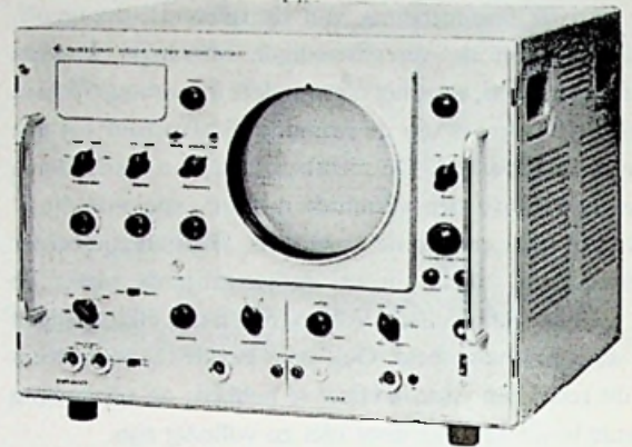
VIDEOSCOPE, TYPE SWOF GROEPLOOPTIJDMETER, TYPE LFM
