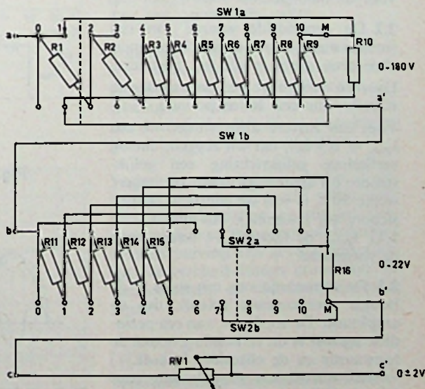
Fig. 8 VOOR AANZICHT SCHAKELDEKKEN ZIE FIG. 7
